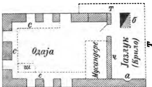
Пресјек горњег боја једне муслиманске куће у Мостару Размјер 1 : 150
