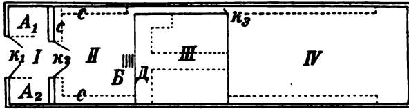
Шематски пресјек једне мусломанске куће у Мостару.
